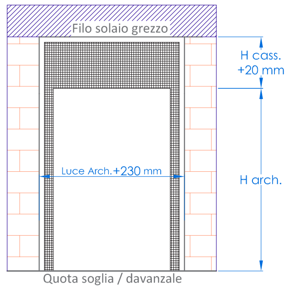
Manovra Motorizzata
